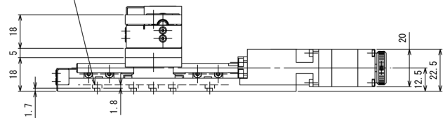
低頭六角穴付きボルト M2.5、長さ6
