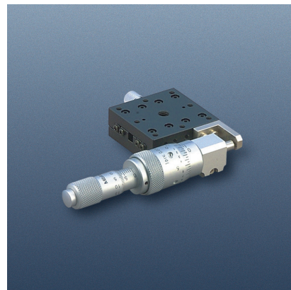
LS-447-R2 逆サイドマイクロ付
