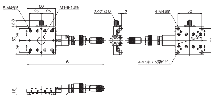
センターマイクロ付(型式末尾-C2)
