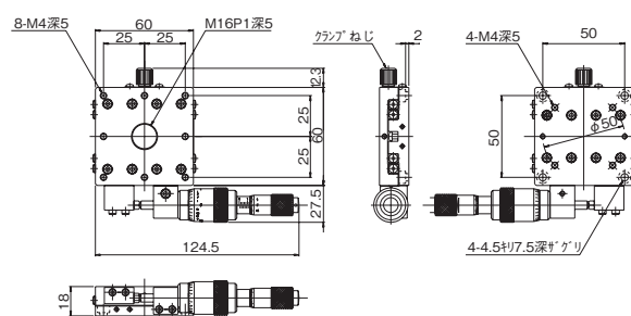
サイドマイクロ付(型式末尾-S2)
