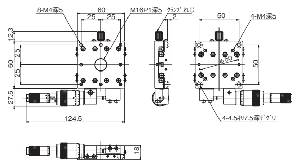
逆サイドマイクロ付(型式末尾-R2)
