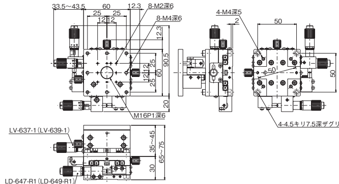
LT-607-R1 (LT-609-R1) X・Yステージ 逆サイドマイクロ付
