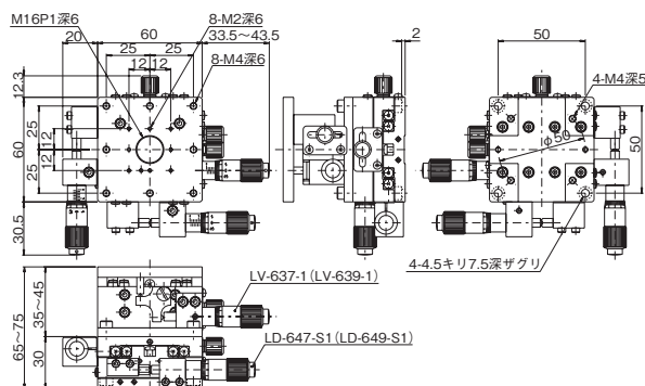
LT-607-S1 (LT-609-S1) X・Yステージ サイドマイクロ付
