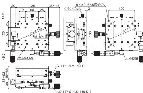
LT-147-S1 (LT-149-S1) X・Yステージ サイドマイクロ付
