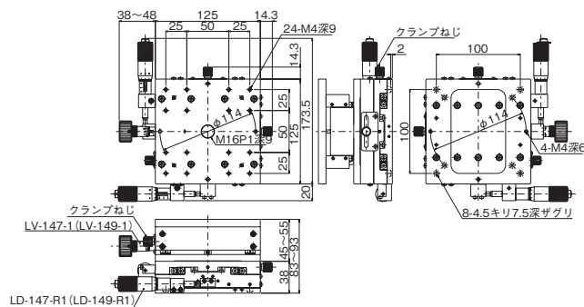
LT-147-R1 (LT-149-R1) X・Yステージ 逆サイドマイクロ付
