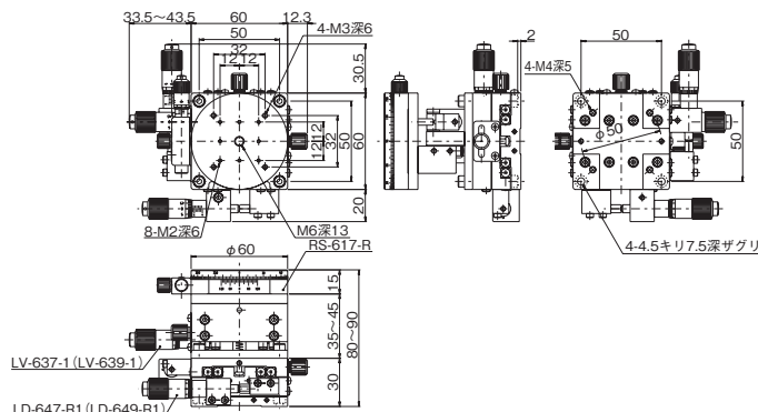
TR-607-R1 (TR-600-R1) X・Yステージ、回転ステージ 逆サイドマイクロ付
