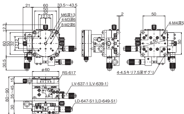
TR-607-S1 (TR-600-S1) X・Yステージ、回転ステージ サイドマイクロ付
