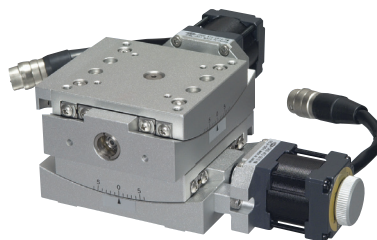
ATD-C612-HM
