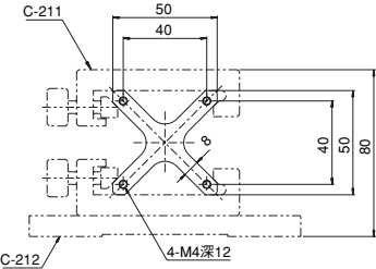
レール、レールキャリアおよびレールスタントの組み合わせ図
