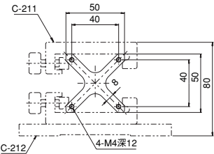
レール、レールキャリアおよびレールスタント'組み合わせ図
