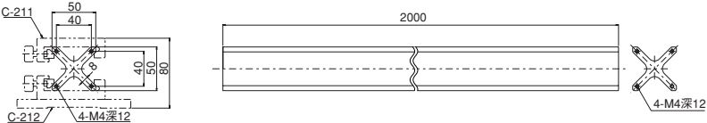
レール、レールキャリアおよびレールスタントの組み合わせ図
