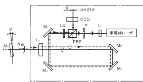
図1 光学系
