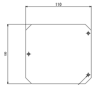
水平調整用ねじ(3ヶ所) 7mmプレート
