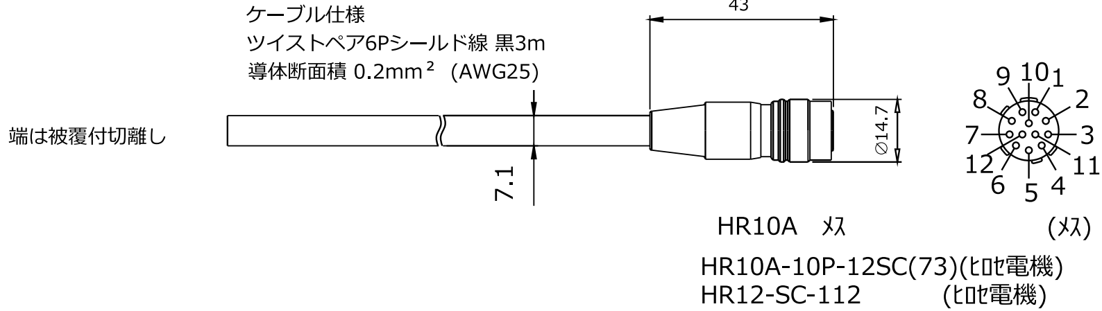
結線仕様図
